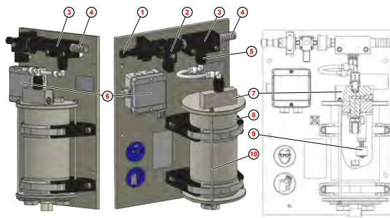
Abb. 5: Aufbau
