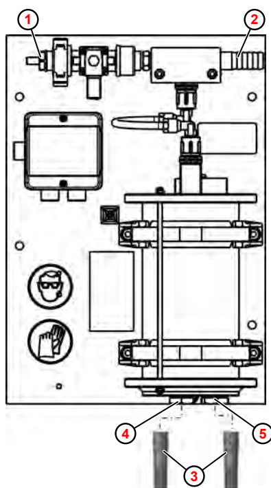
Fig. 9 : Installation hydraulique
