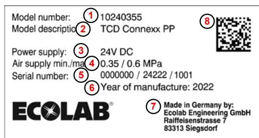
Fig. 17 : Plaque signalétique
