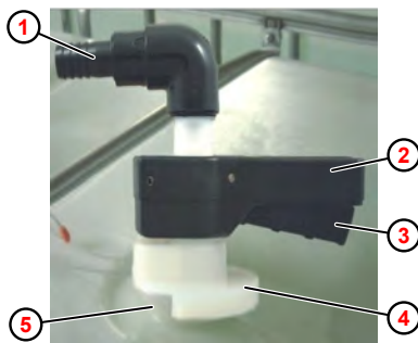
Abb. 3: „Click & Plug“-Anschlusskupplung
