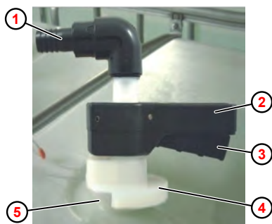
Fig. 3 : Dispositif d'accouplement « Click & Plug »
