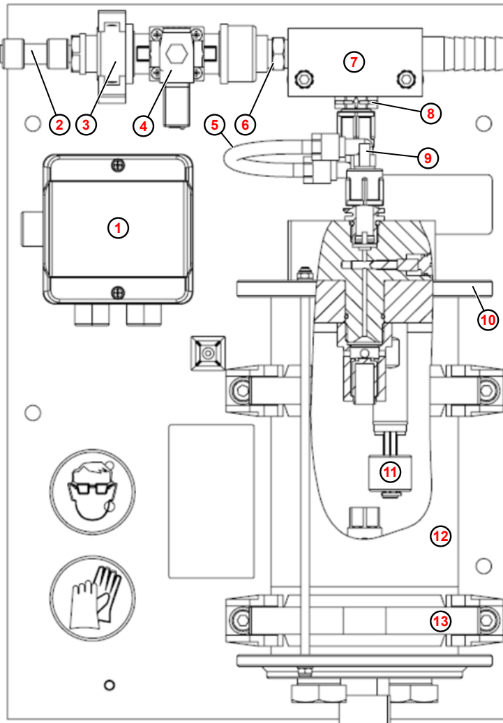
Abb. 16: Ersatzteile
