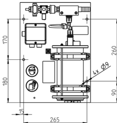
Fig. 7 : Montage mural Connexx TCD PP
