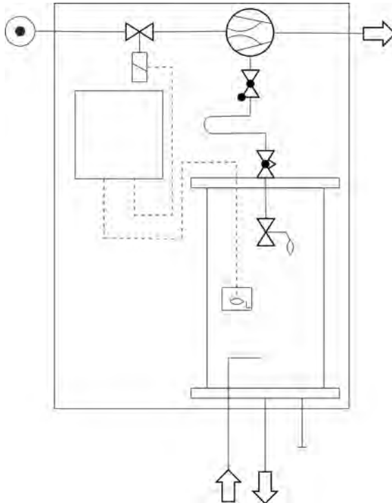
Abb. 1: Funktionsschema
